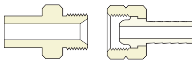
Connection 024 0.875" – 14UNF RH EXT.
