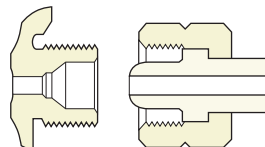
Connection 410 0.85" – 14NGO LH EXT.
